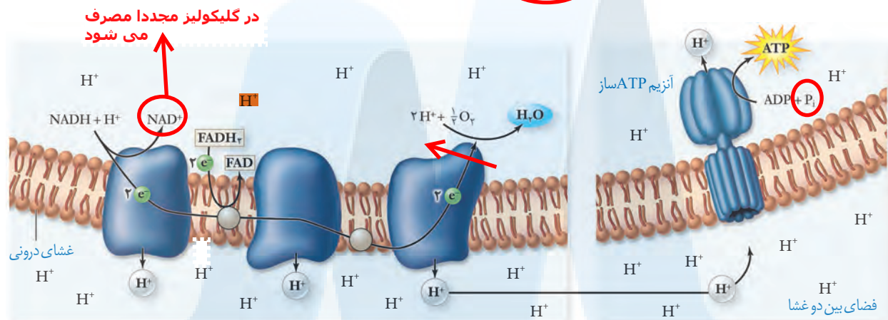
شکل ۸- زنجیره انتقال الکترون در راکتیزه و تشکیل ATP
