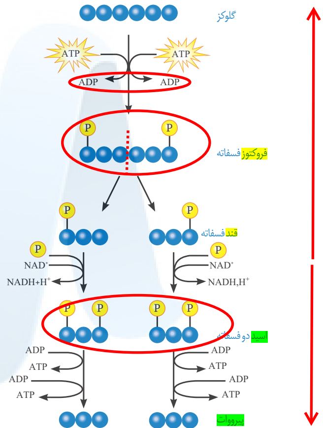
شکل ۴- مراحل قندکافت
