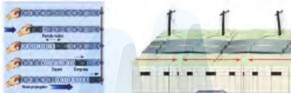
شکل ۳-۶: موج P
