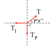
۲. گزینه ۳ با استفاده از قضیه ی سینوس ها:
